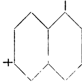
Bad. Anilin- u. Sodafabr. D. R.-Patent 57 910. Pat.-Anm. 9568 Kalle & Co.
